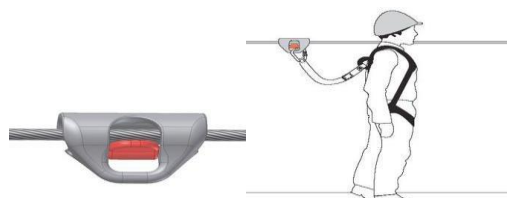
Fig. 9 Orientació correcta del carro en la línia
