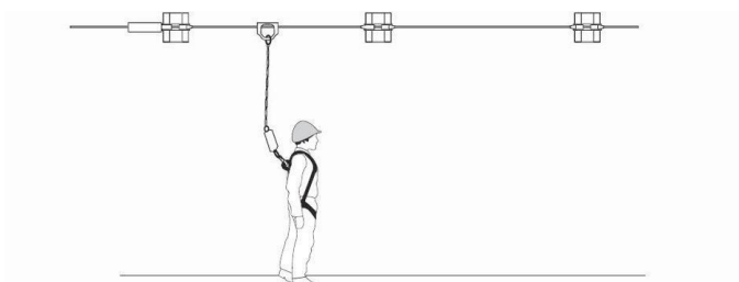
Fig.1 Usuari assegurat a la línia de vida
