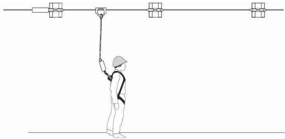
Fig.1 Usuario asegurado a la línea de vida
