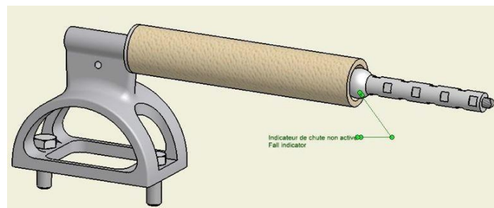
Fig. 2 Indicador de caída no activado
