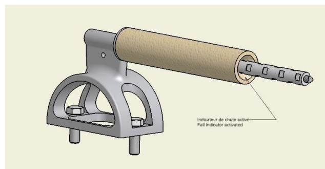
Fig.3 Indicador de caída activado
